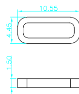
防水圈图示
